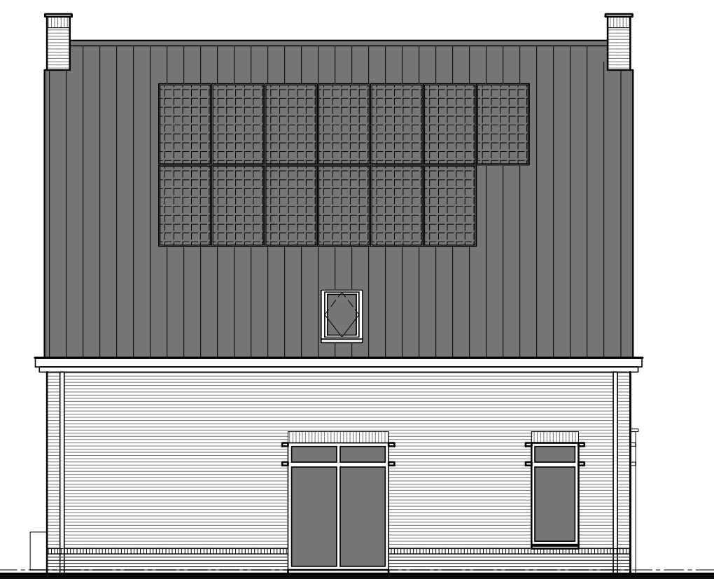
Linkerzijgevel bwnr. 5 schaal 1:100
