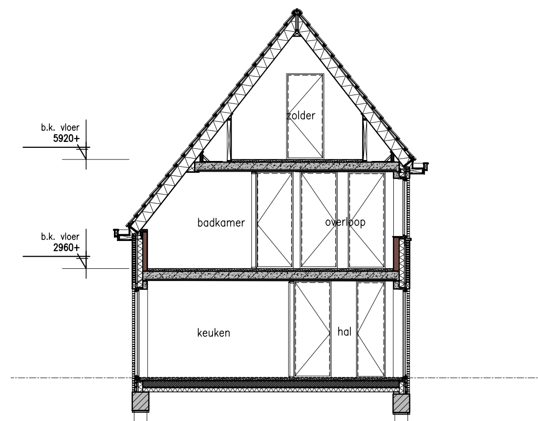
Doorsnede A-A
