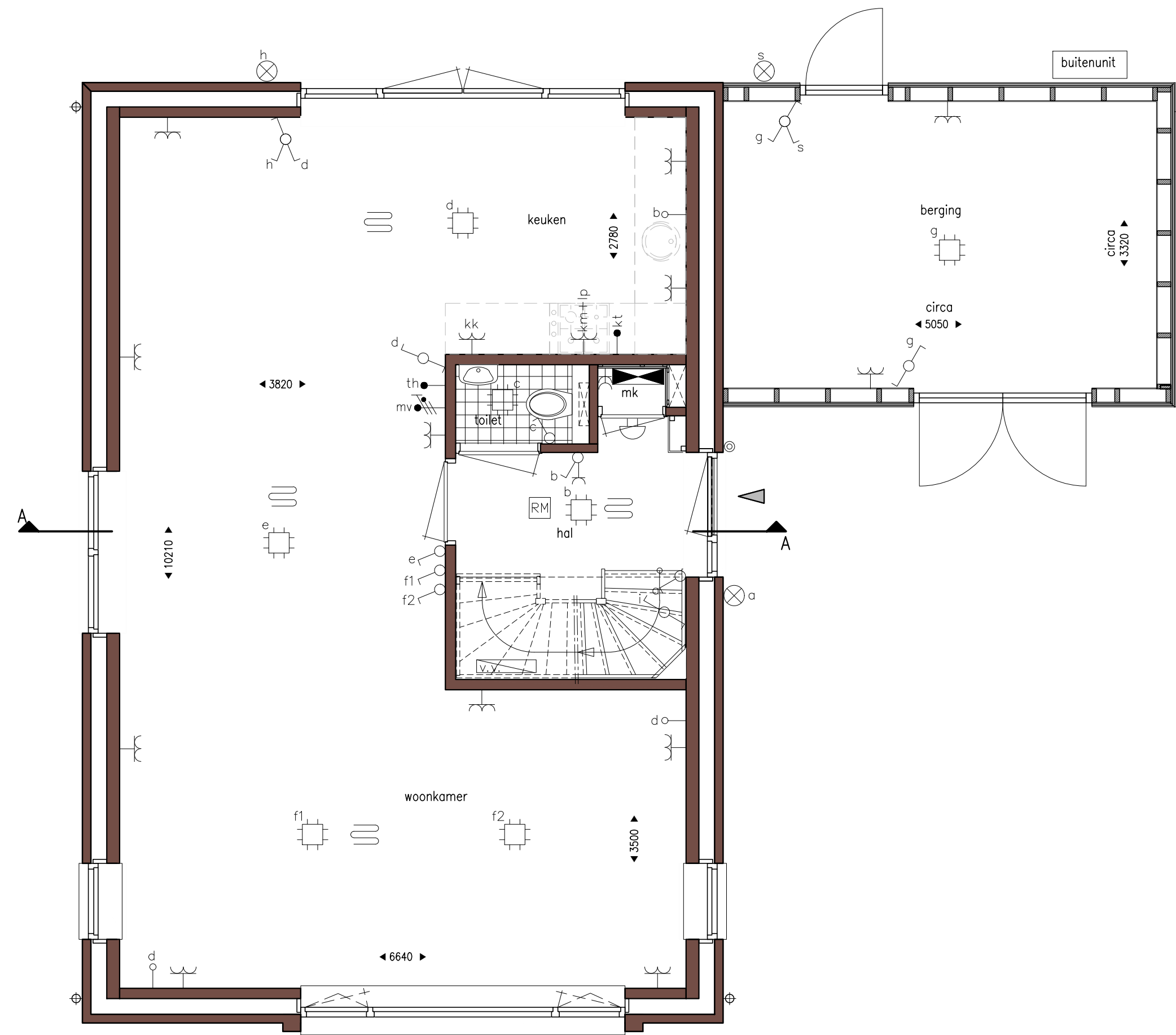
Begane grond Bouwnr. 05 schaal 1:50
