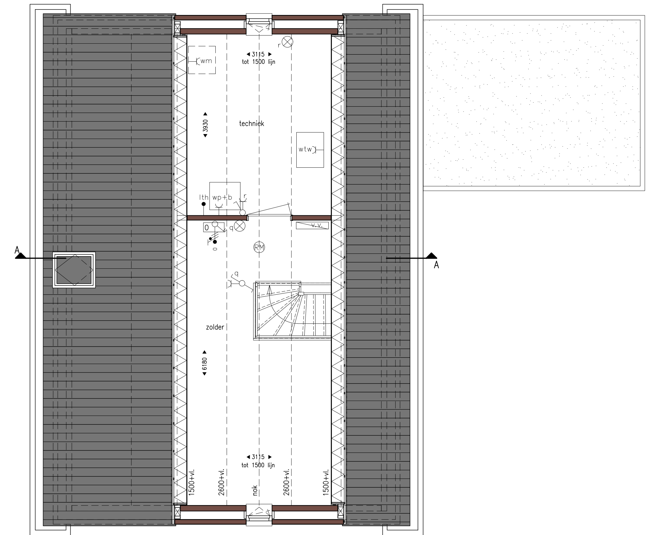
2e verdieping Bouwnr. 05 schaal 1:50
