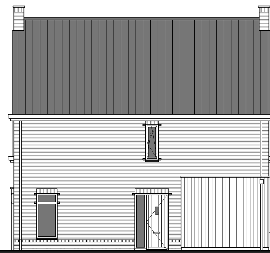
Rechterzijgevel bwnr. 5 schaal 1:100
