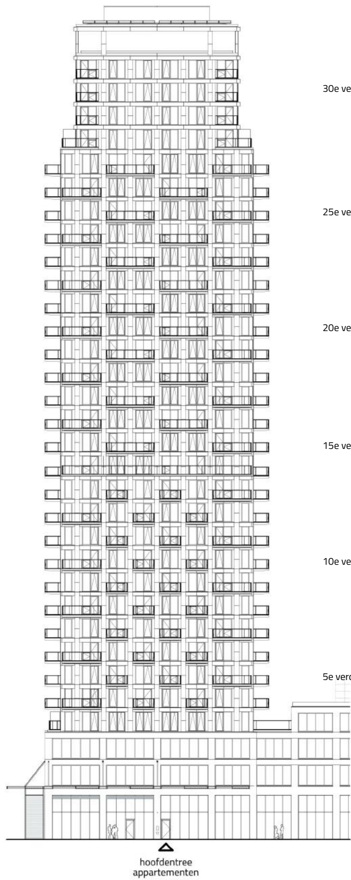
Zuidoost gevel
