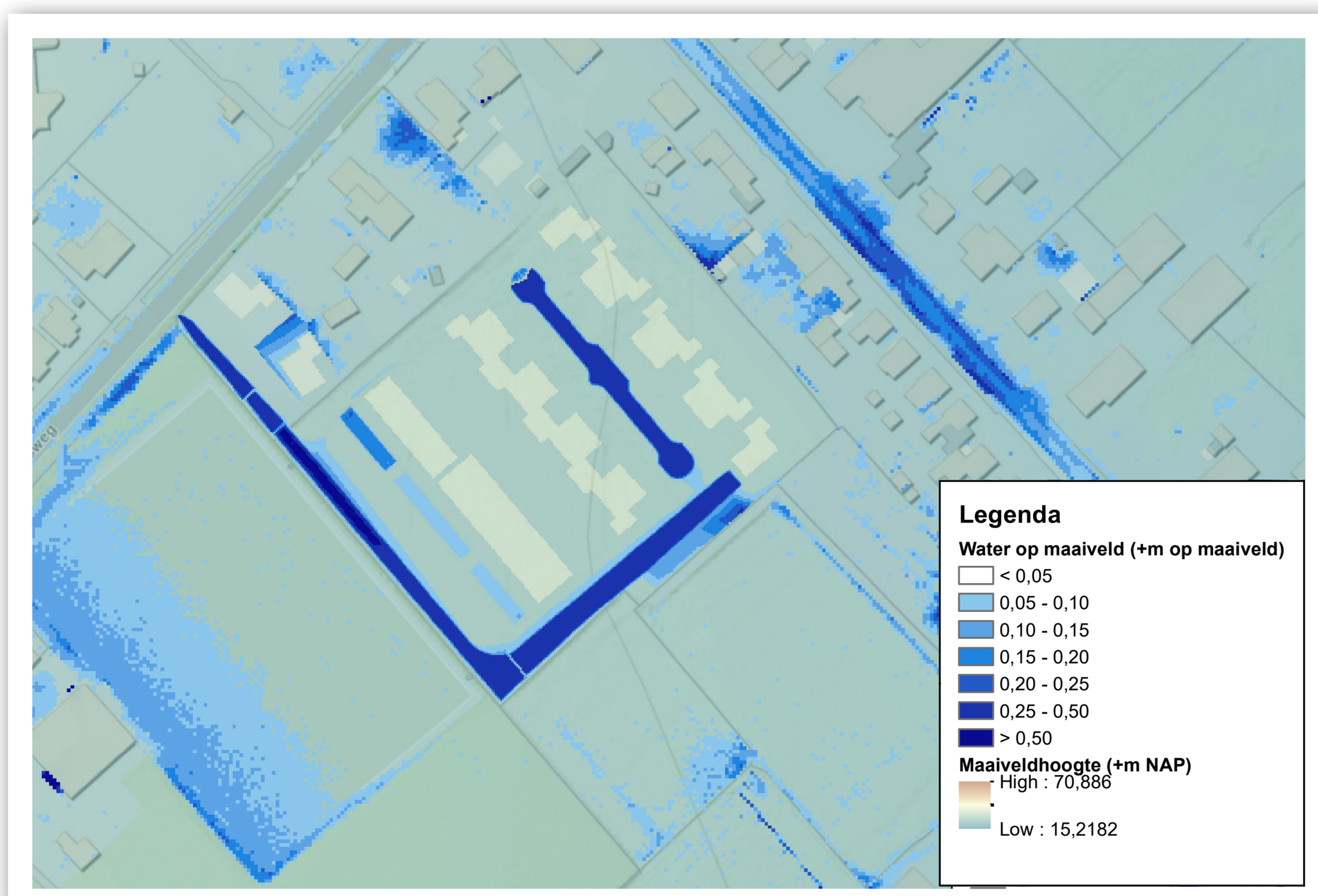
Woningbouwproject Antoniushof mét impact van de omgeving inclusief maatregelen stroombanenplan gemeente/waterschap Piekmoment: 50 minuten na aanvang van de 30 mei 2016 bui (60 mm neerslag in 2 uur tijd)
