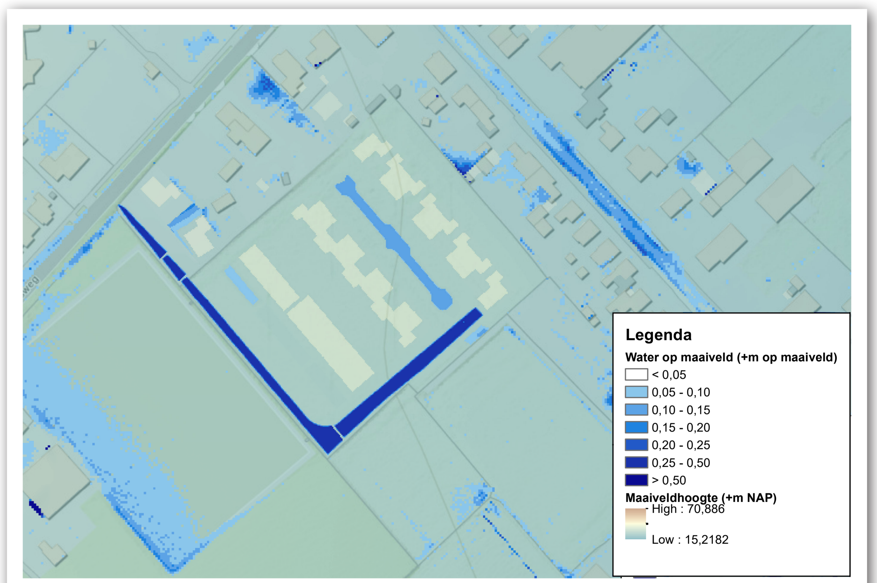
Woningbouwproject Antoniushof mét impact van de omgeving inclusief maatregelen stroombanenplan gemeente/waterschap Moment 1 uur na het piekmoment van de 30 mei 2016 bui (60 mm neerslag in 2 uur tijd)
