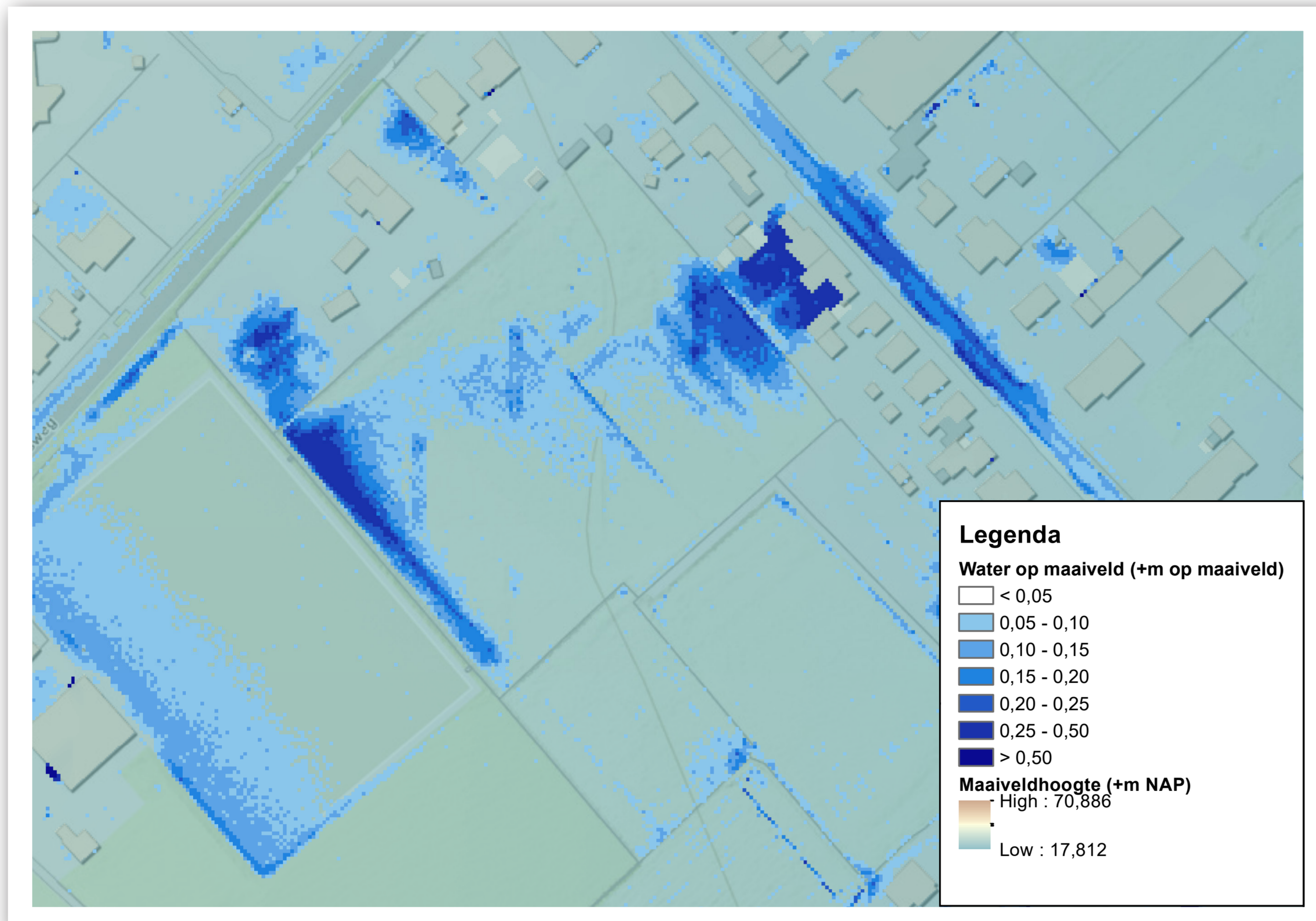
Huidige situatie (zonder Antoniushof) maar inclusief maatregelen stroombanenplan gemeente/waterschap Piekmoment: 50 minuten na aanvang van de 30 mei 2016 bui (60 mm neerslag in 2 uur tijd)
