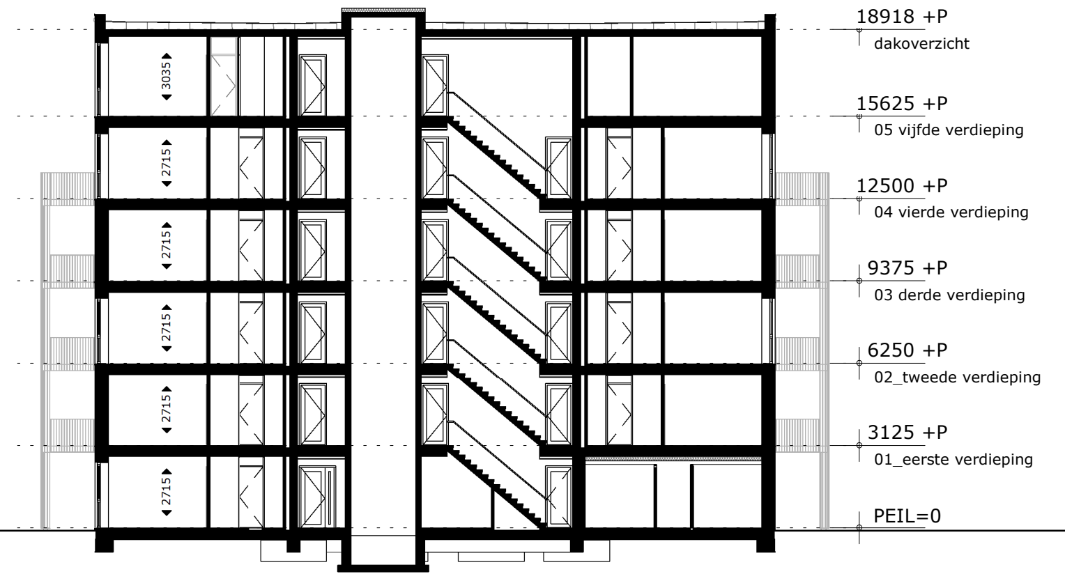
doorsnede B-B
