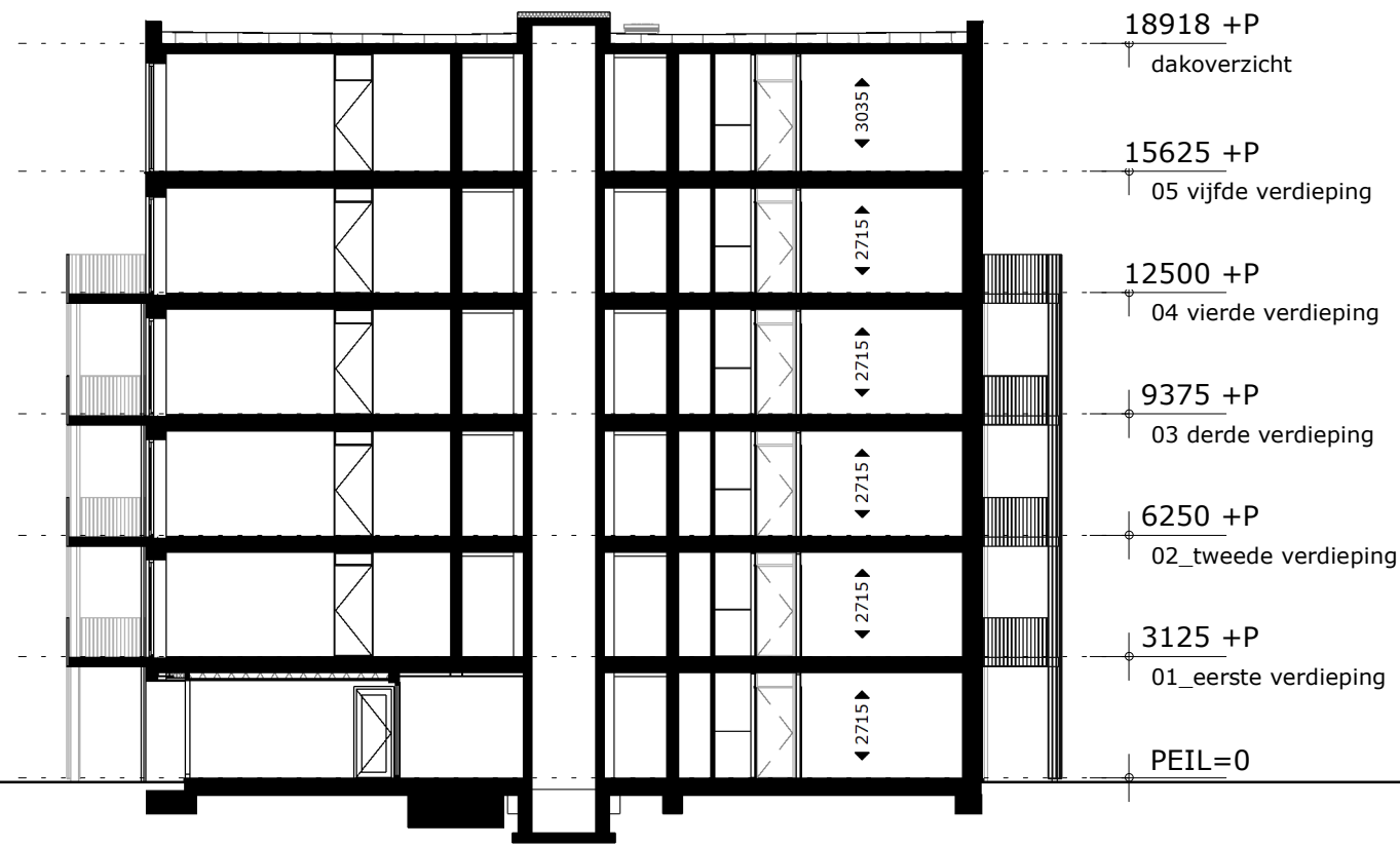
doorsnede A-A
