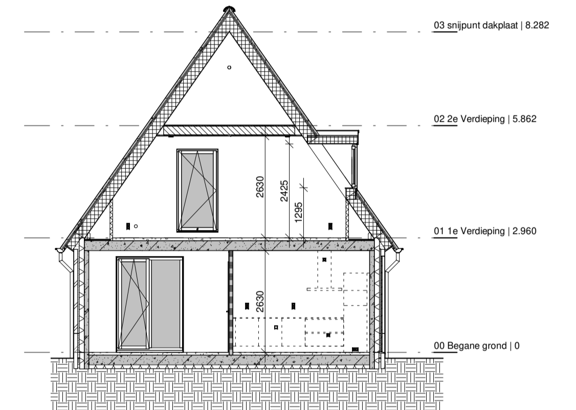
Doorsnede A
