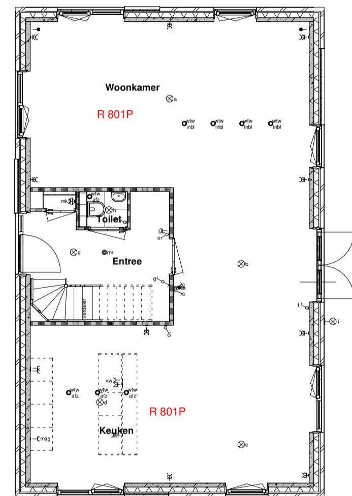
Begane grond
