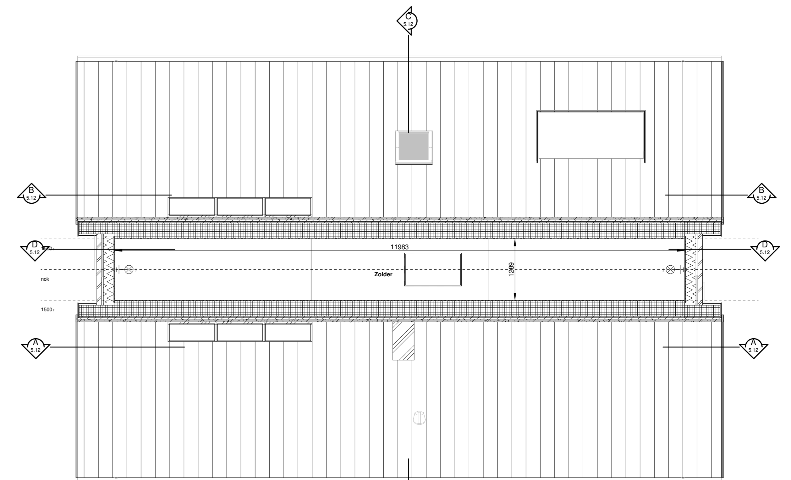
Vliering Schaal: 1 : 50
