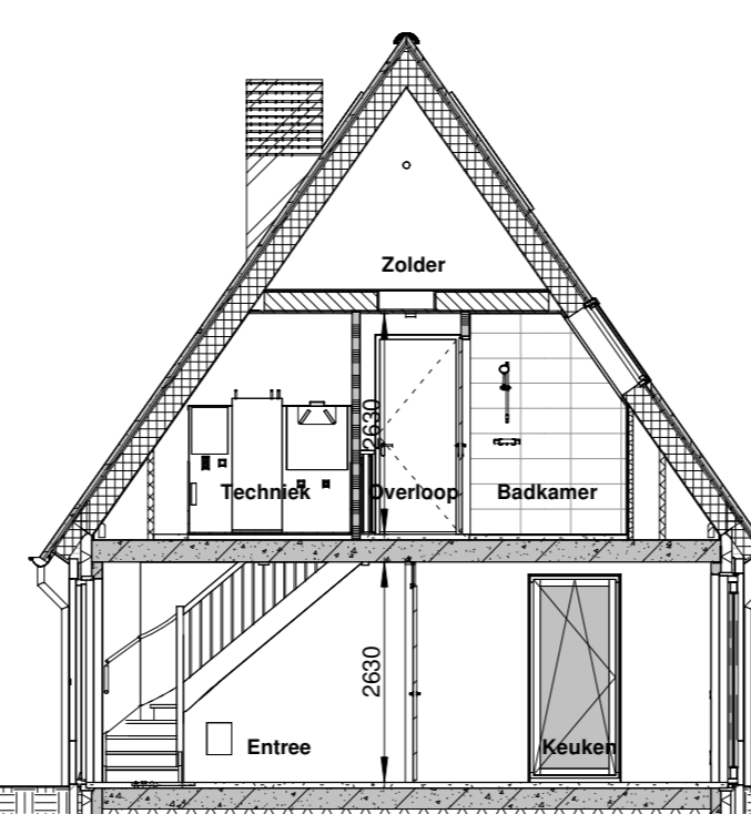
Doorsnede CC Schaal: 1 : 100
