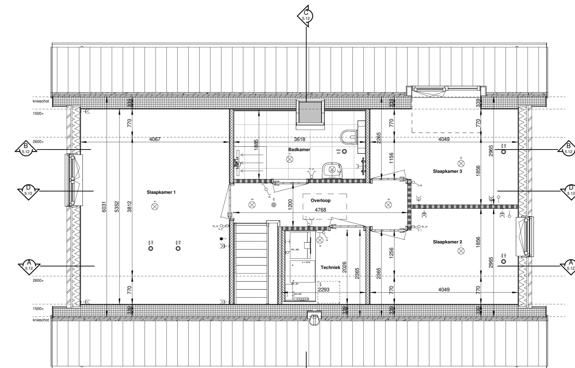
Verdieping 1 Schaal: 1 : 50
