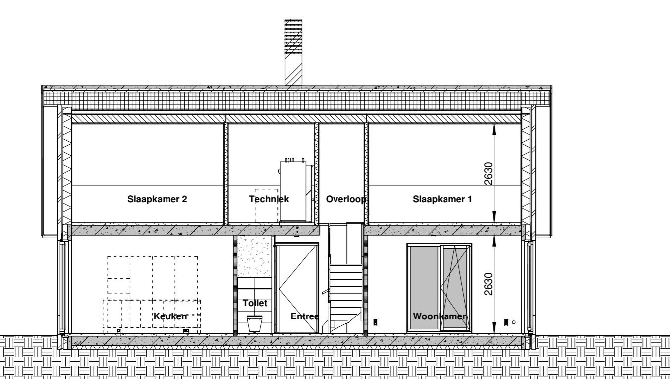
Doorsnede AA Schaal: 1 : 100
