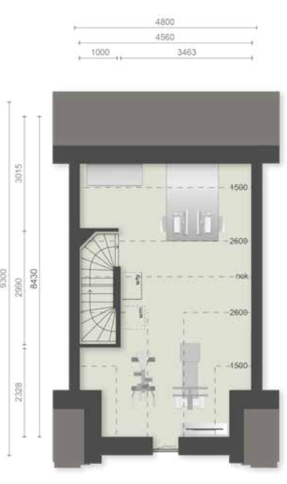
TWEDE VERDIEPING
