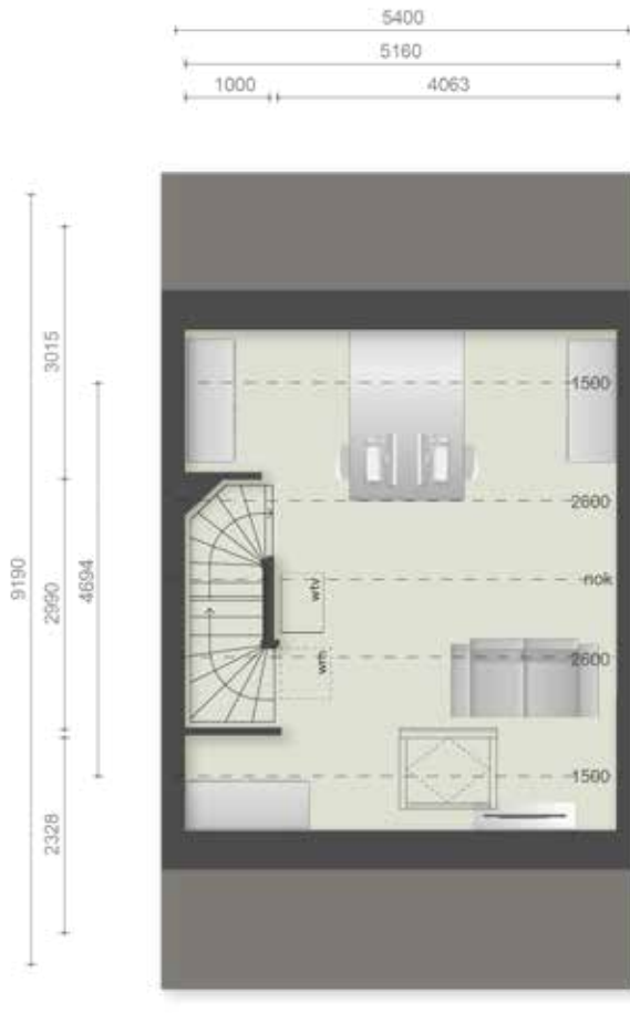
TWEEDE VERDIEPING
