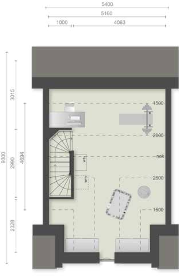
TWEEDE VERDIEPING
