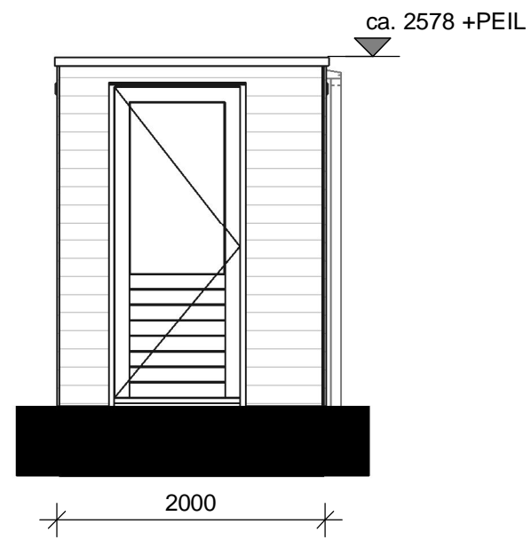
rechter zijgevel 1:50
