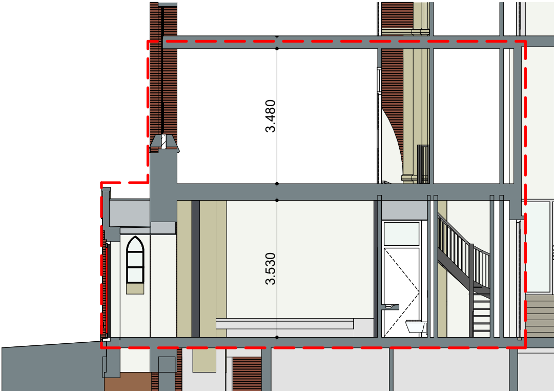
doorsnede
