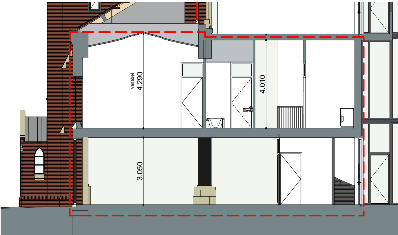
doorsnede
