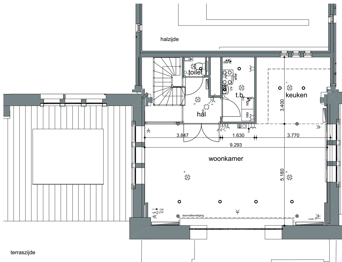
3e verdieping
