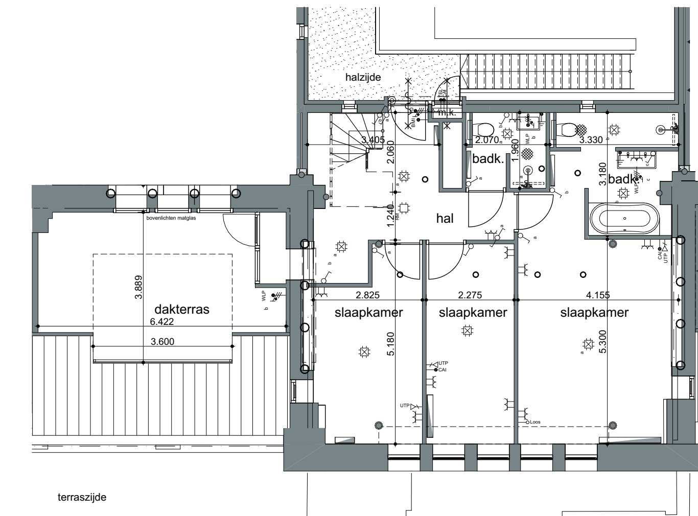
2e verdieping
