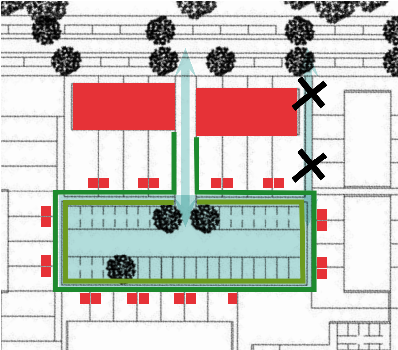
Indeling parkeerhof A (4 zijden bebouwd) Entree tussen bebouwing (niet langs achtertuin), omgang hagen en bijgebouwen Fase 1
