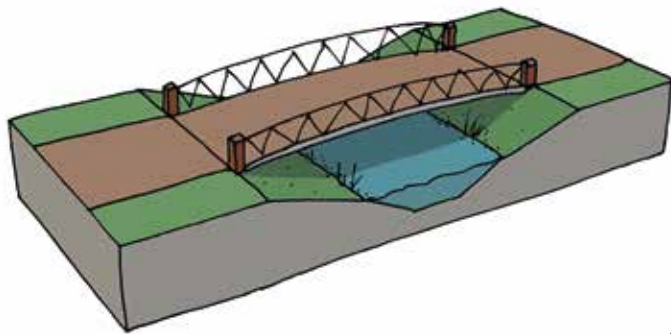
1A Gemetselde poeren + doorlopend talud
