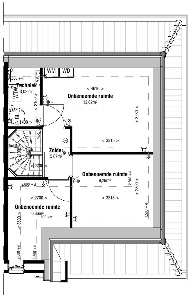
B 007 2e verdieping extra indeling type D/E
