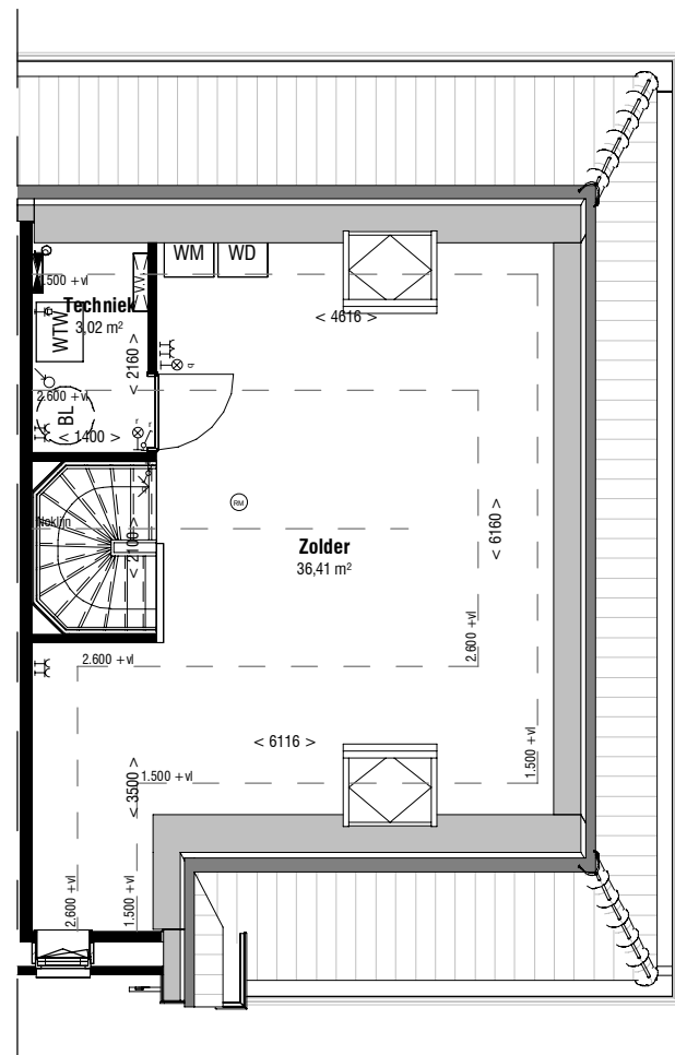
R 070 F-A-1 Dakraam voor of achtergevel
