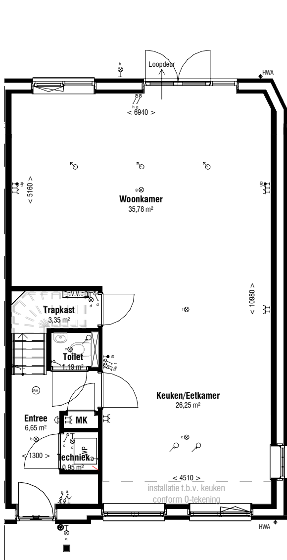
R 009 Achterruitbouw van 1200mm
