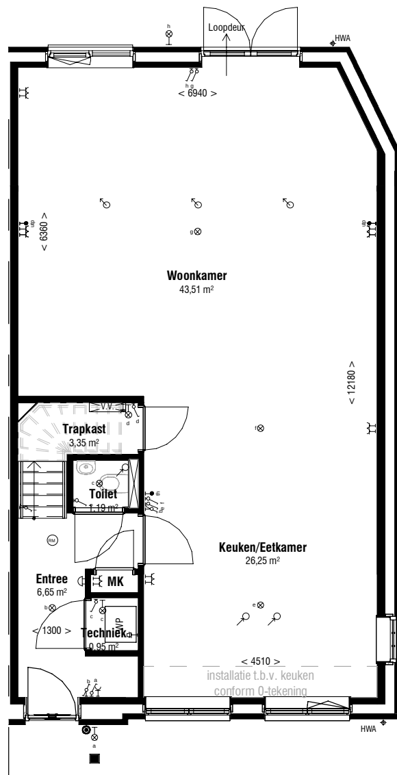
R 018 Achterruitbouw van 2400mm
