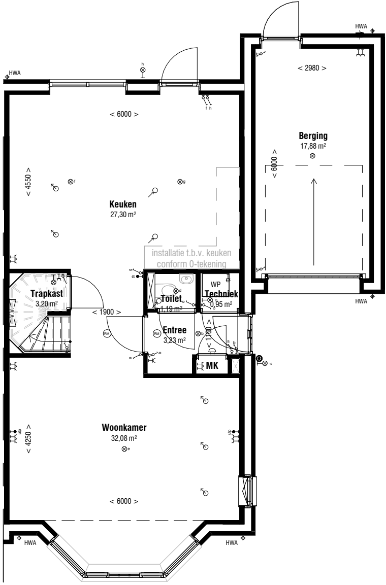
R 007 Achteruitbouw van 1200mm
