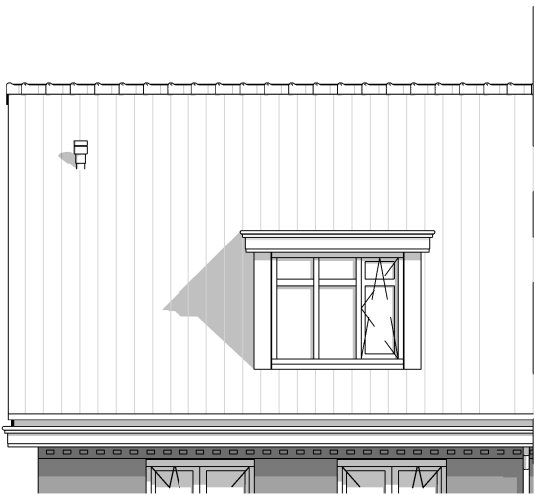
R 061 A Dakkapel type D/E/F achtergevel
