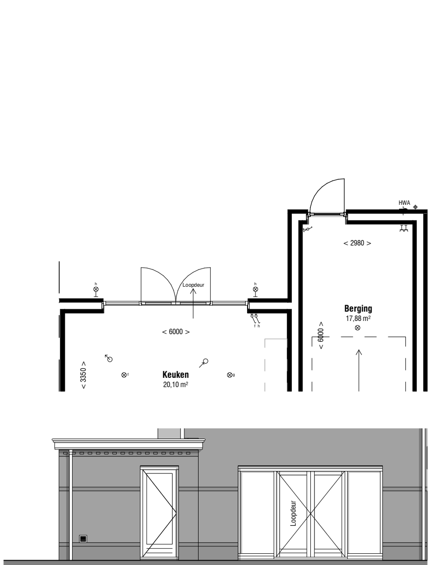
R 094 H Dubbele tuindeuren met zijlichten
