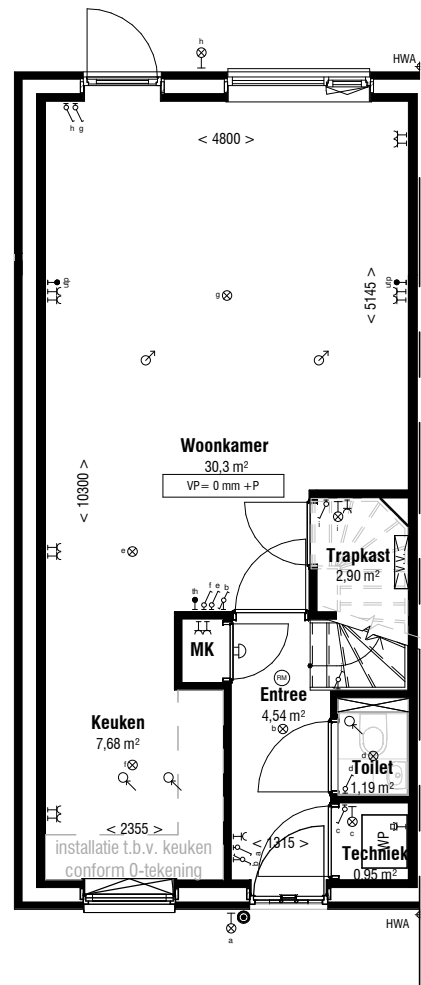
R 012 Achteruitbouw van 2400mm
