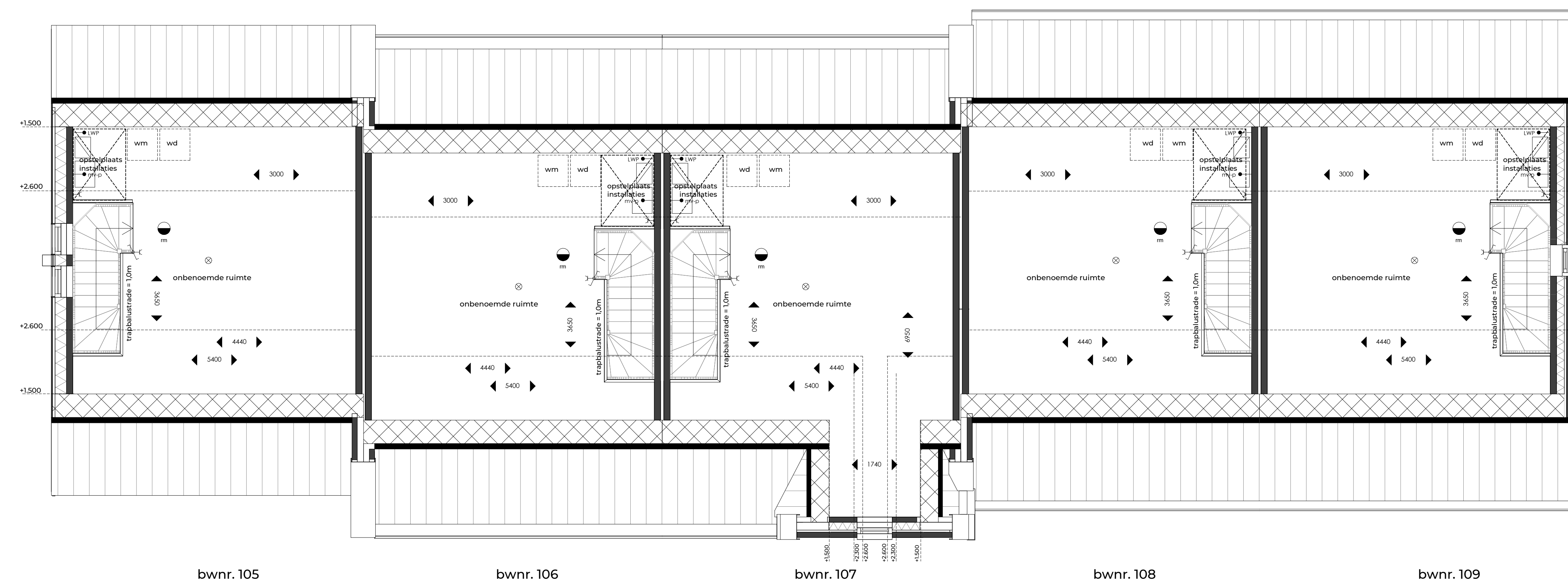
2e verdieping 1:50
