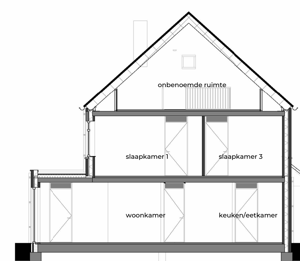
doorsnede C-C 1:100
