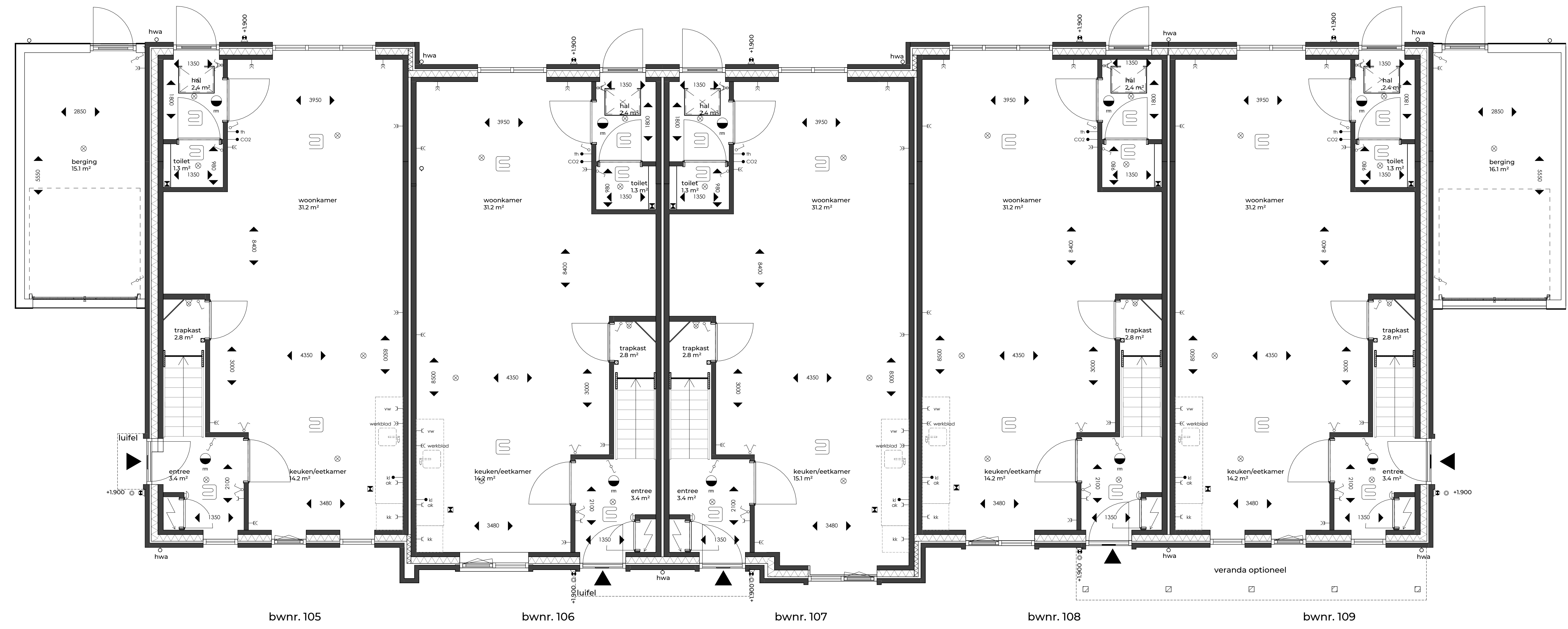
begane grond 1:50
