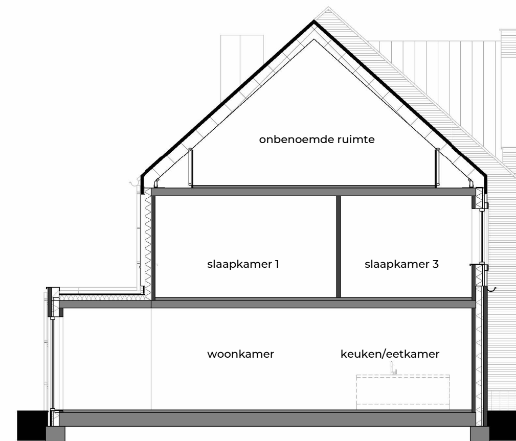
doorsnede A-A 1:100
