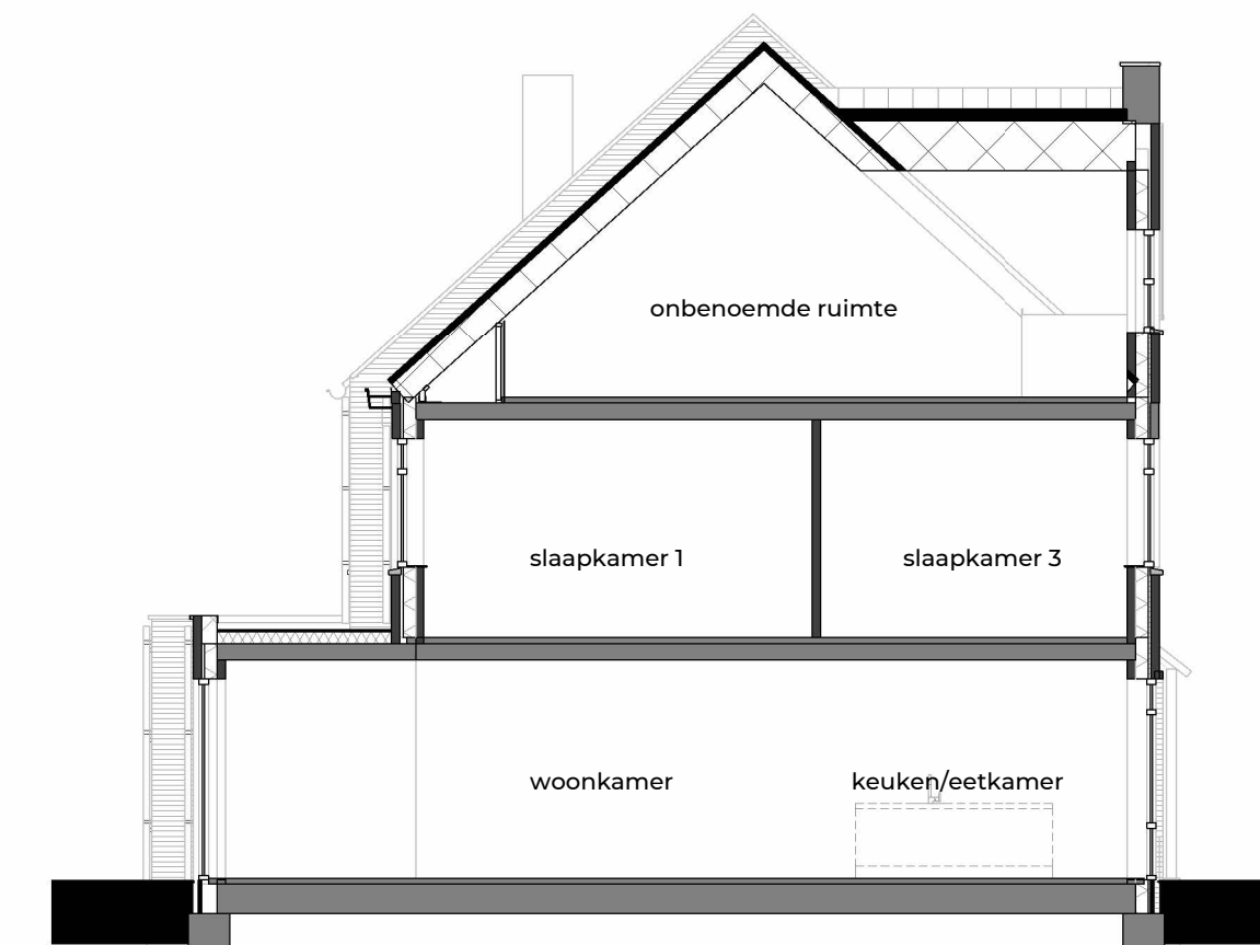
doorsnede B-B 1:100
