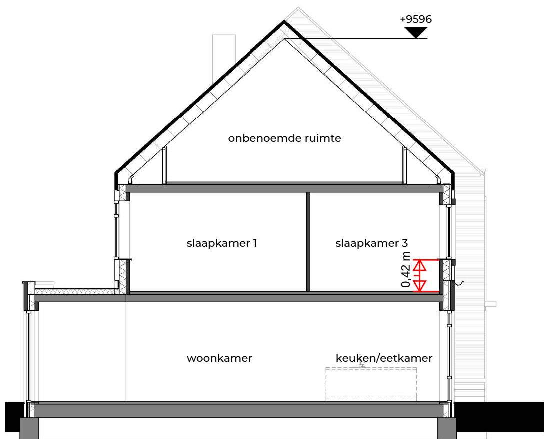
doorsnede A-A 1:100
