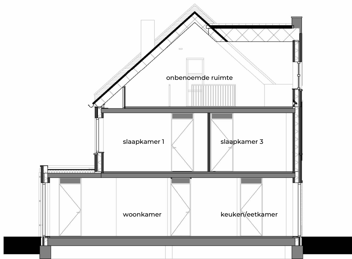
doorsnede C-C 1:100
