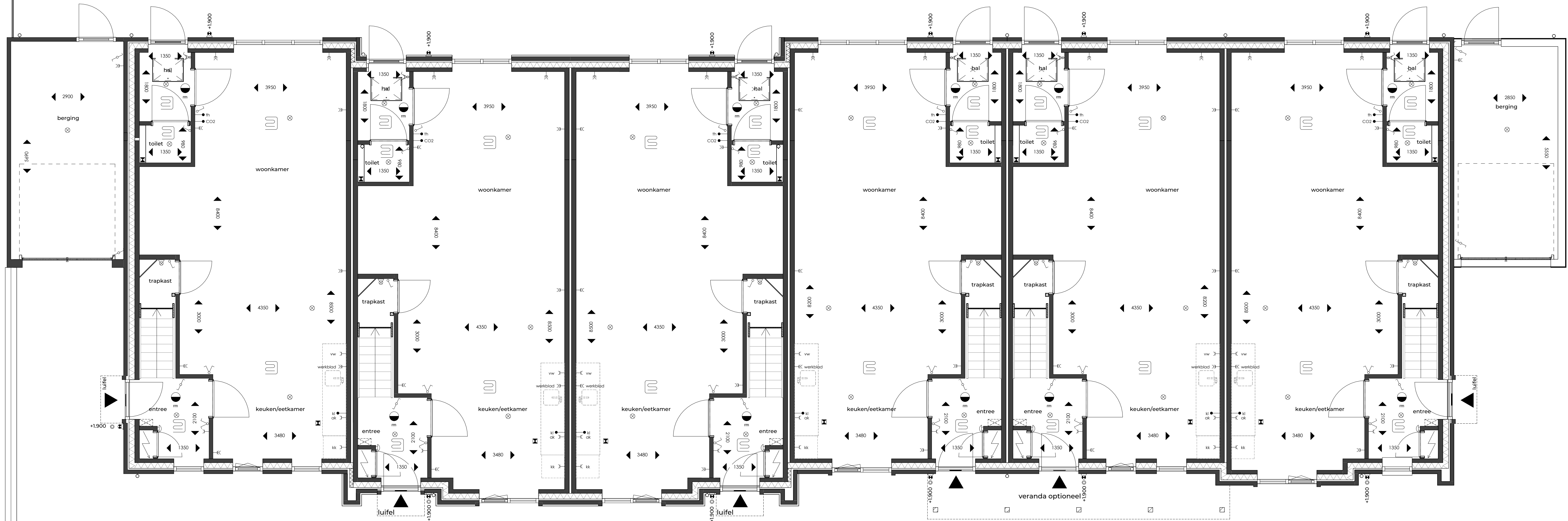
begane grond 1:50
