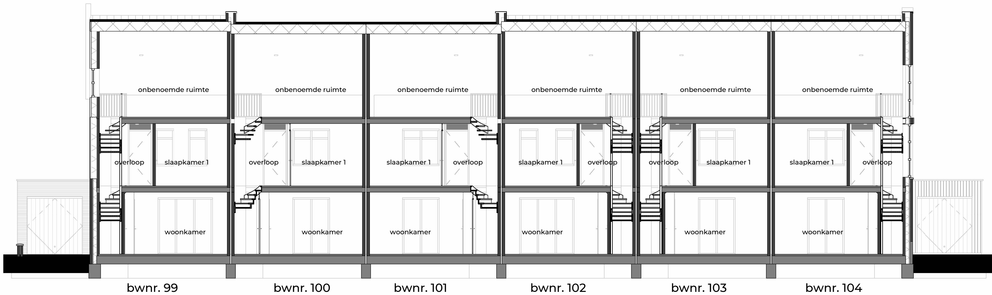
doorsnede D-D 1:100
