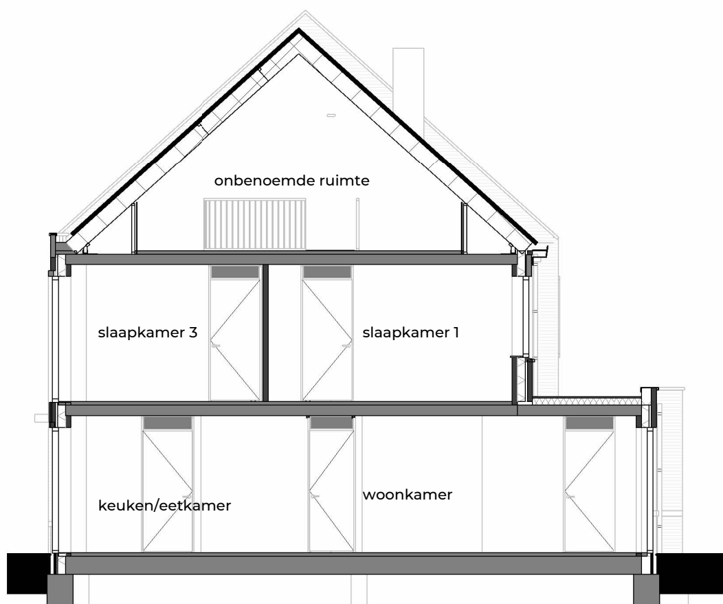
doorsnede B-B 1:100
