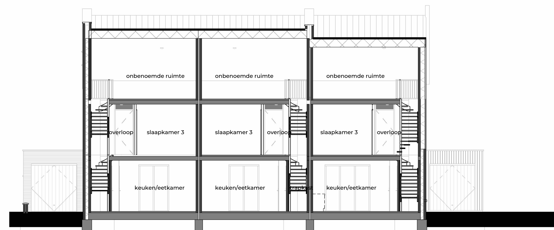
doorsnede B-B 1:100
