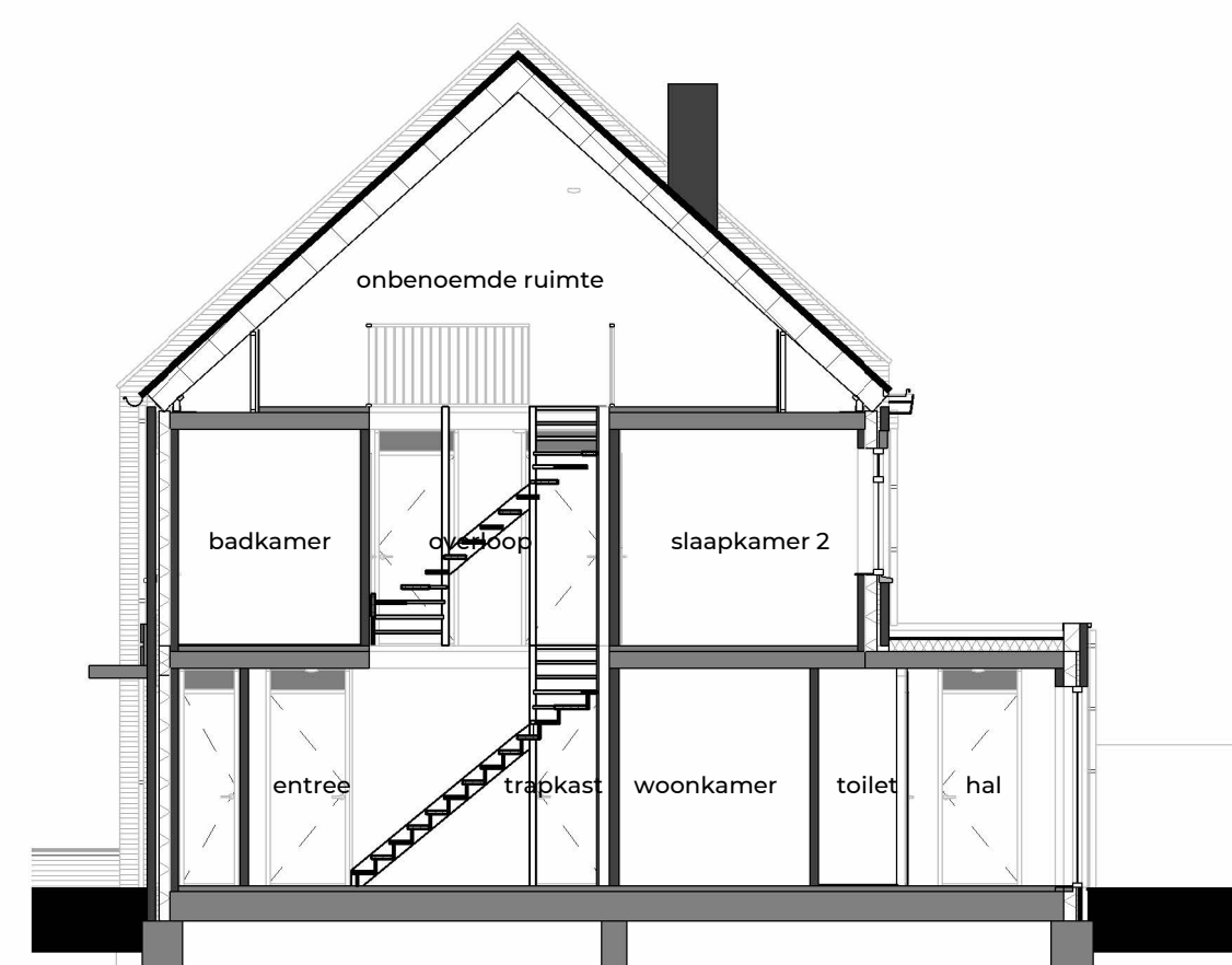
doorsnede A-A 1:100
