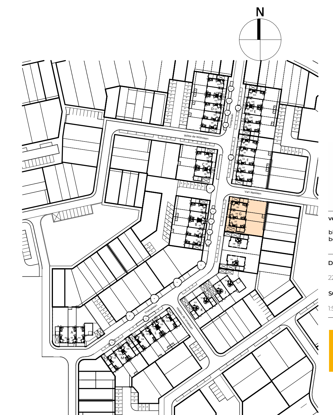
situatie 1:1500
